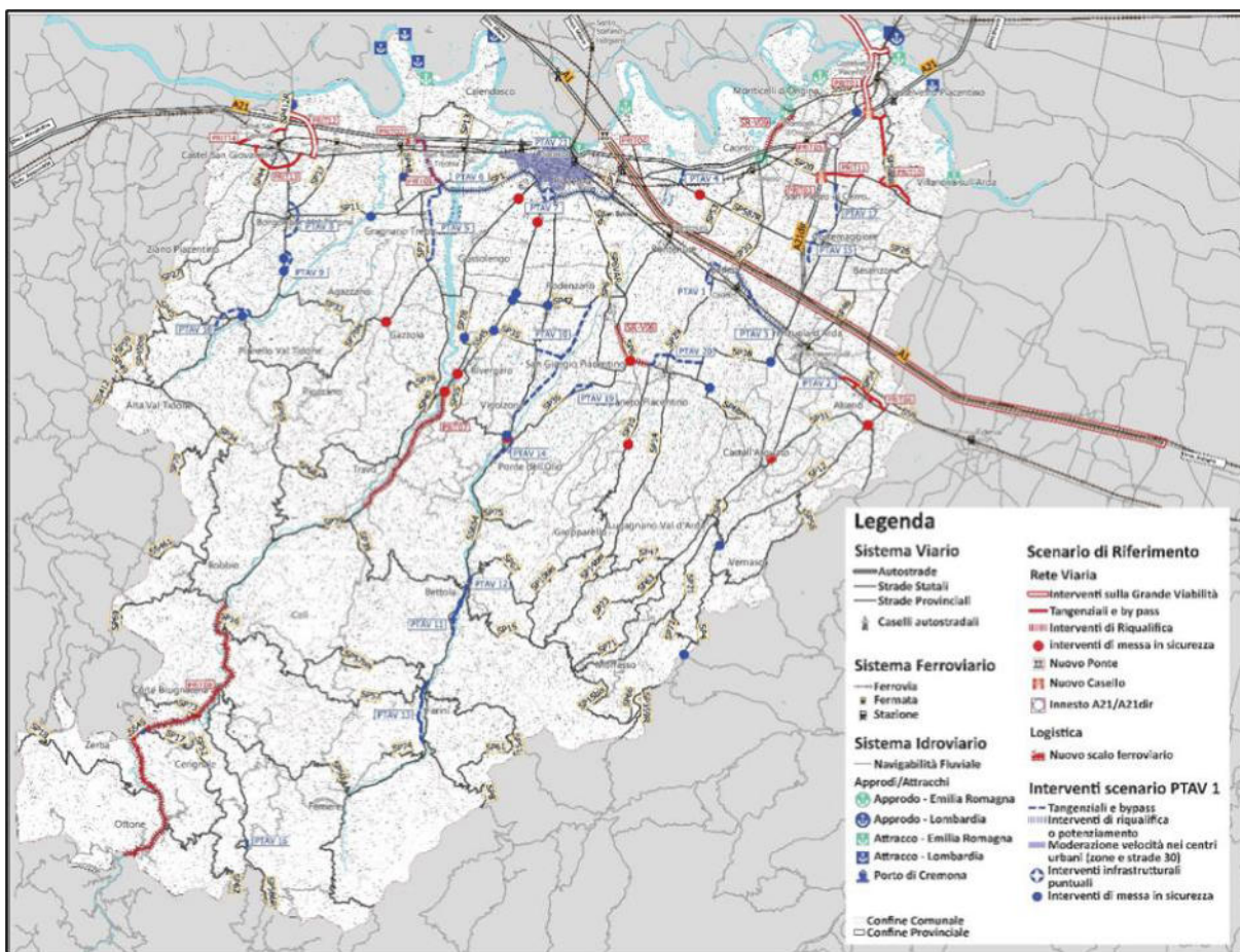
Figura 3.3.5 – Scenario PTAV1 + Scenario di Riferimento: interventi infrastrutturali.
