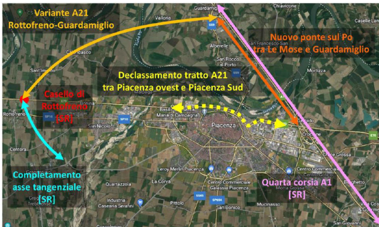
Figura 3.3.4 – Sistema complesso di interconnessione A21-A1-SS9, schema degli interventi.
