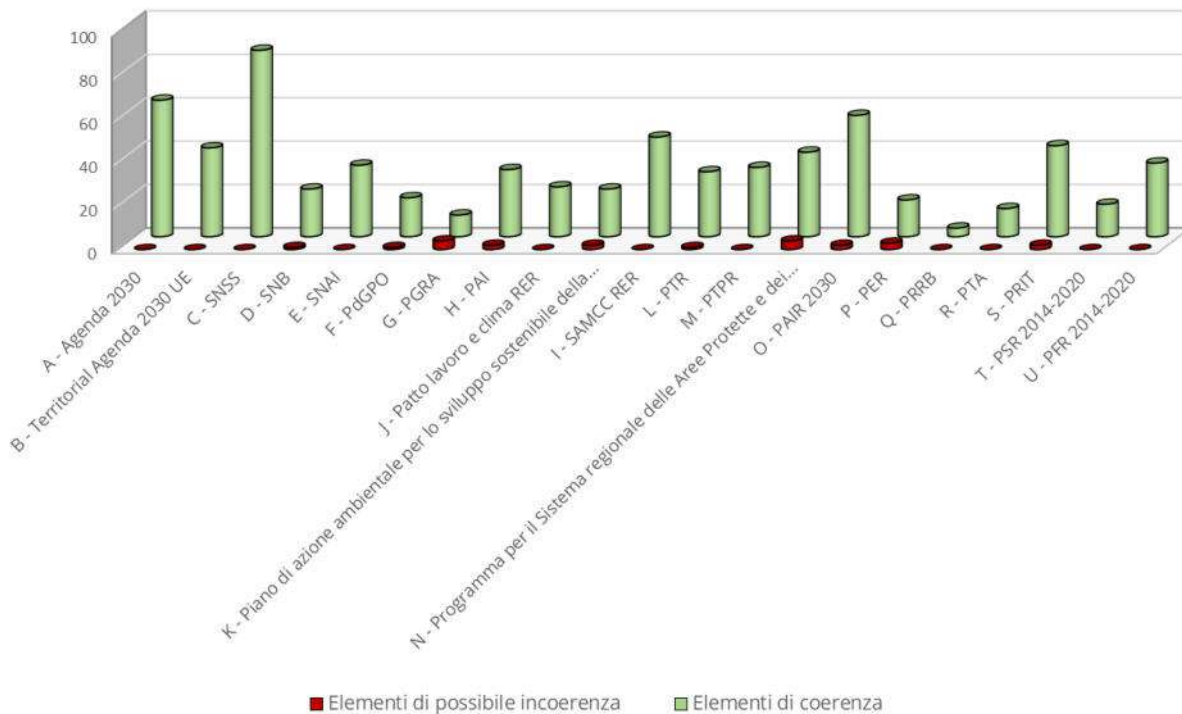
Figura 2.2.2 – Possibili effetti degli Obiettivi Specifici di Piano rispetto agli obiettivi di rango internazionale, nazionale e regionale (Allegato 2.B).
